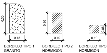
DETALLE BORDILLOS ESCALA 1:10
