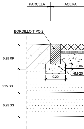
DETALLE_TIPO ESCALA 1:10
