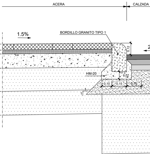
DETALLE_TIPO ESCALA 1:10
