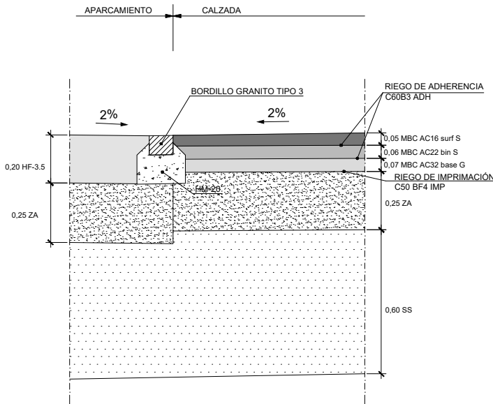
DETALLE_TIPO ESCALA 1:10
