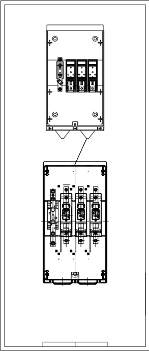
DETALLE SECCIONAMIENTO Y C.G.P.
