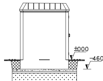
VISTA POR "C"
