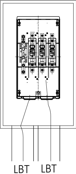
DETALLE SECCIONAMIENTO
