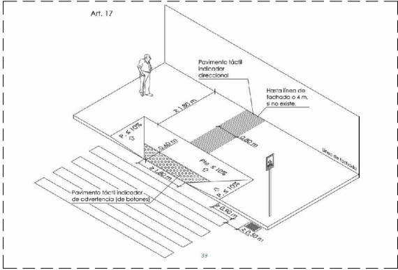
DETALLE VADO D>1,80 m S/E
