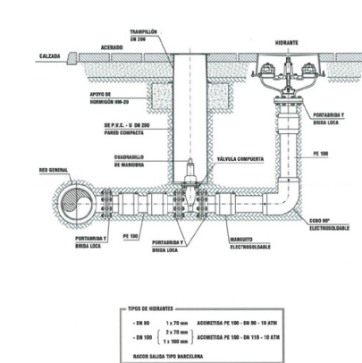
DETALLE DE HIDRANTE
