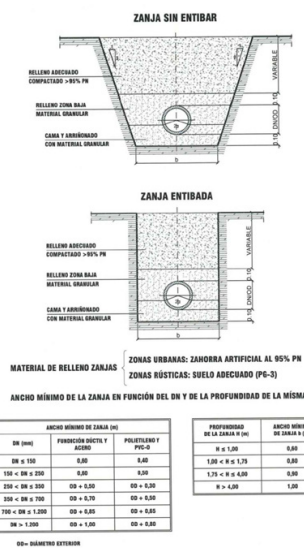
SECCIONES TIPO DE ZANJAS PARA CANALIZACIONES ABASTECIMIENTO
