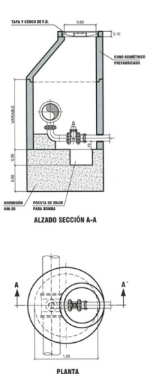
DETALLE DE DESAGÜE EN POZO O ARQUETA
