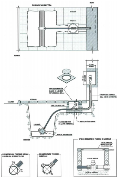
DETALLE DE ACOMETIDA INDIVIDUAL
