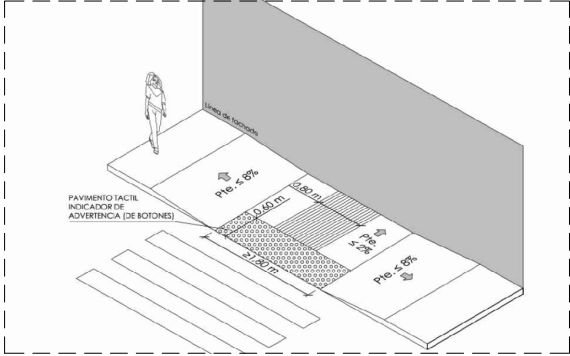
DETALLE VADO D<1,80 m S/E
