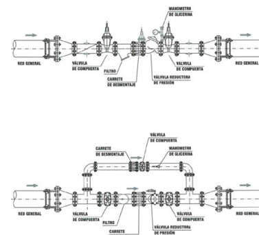
DETALLE DE VÁLVULA REDUCTORA DE PRESIÓN
