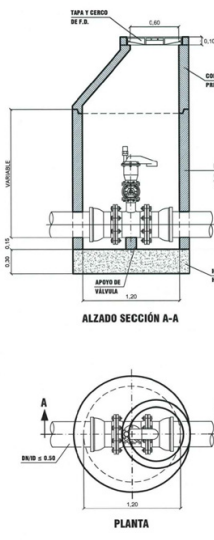
DETALLE DE VENTOSA EN POZO O ARQUETA
