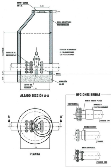
DETALLE DE VÁLVULA DE COMPUERTA EN POZO O ARQUETA
