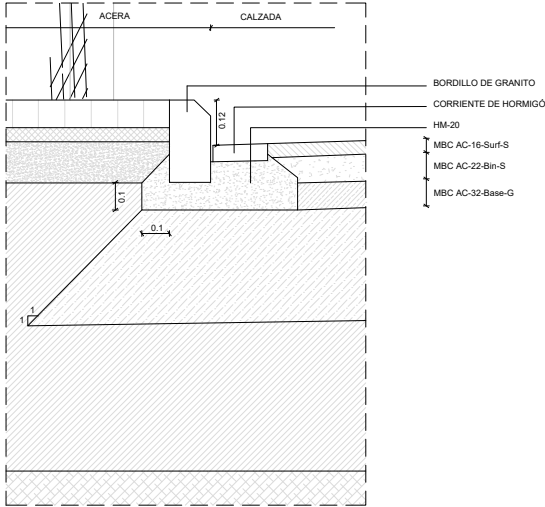
DETALLE BORDILLO E 1:25
