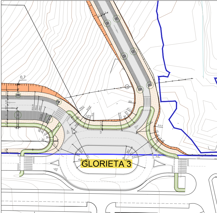
ACCESO A GLORIETA EN C/ BATALLA DEL SALADO
