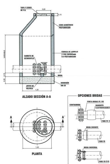
DETALLE DE VÁLVULA DE MARIPOSA EN POZO O ARQUETA
