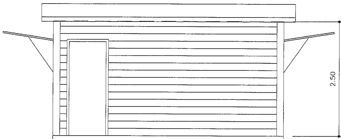
ALZADO POSTERIOR
