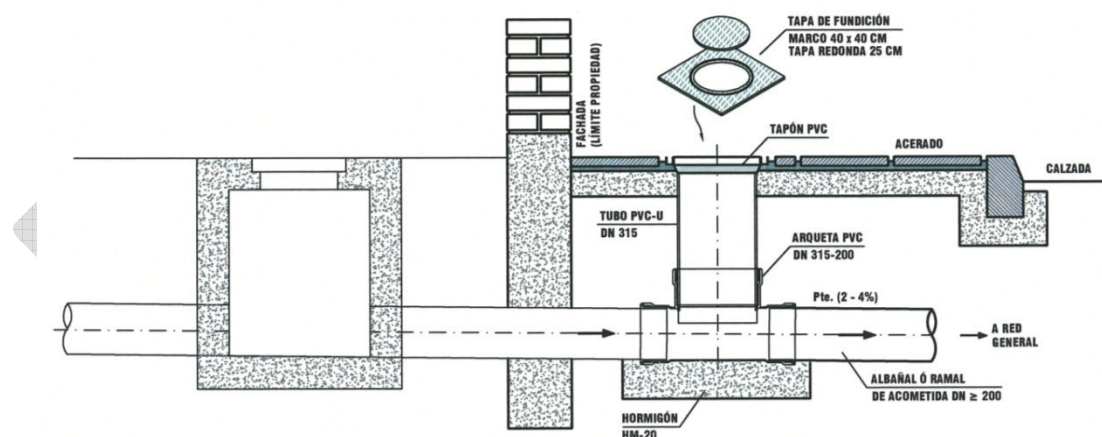
Figura III-2. Edificación sin sótano
