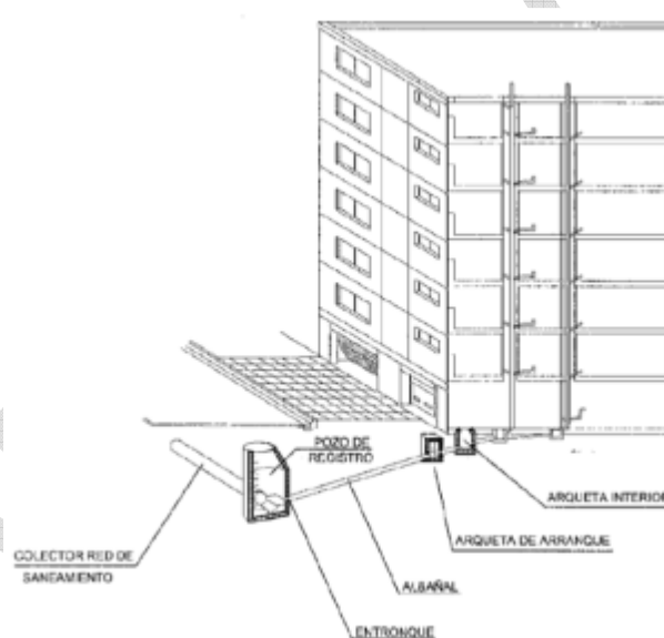
Figura III-1. Componentes de una acometida
