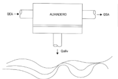
Esquema IV-6. Caudales en los aliviaderos
