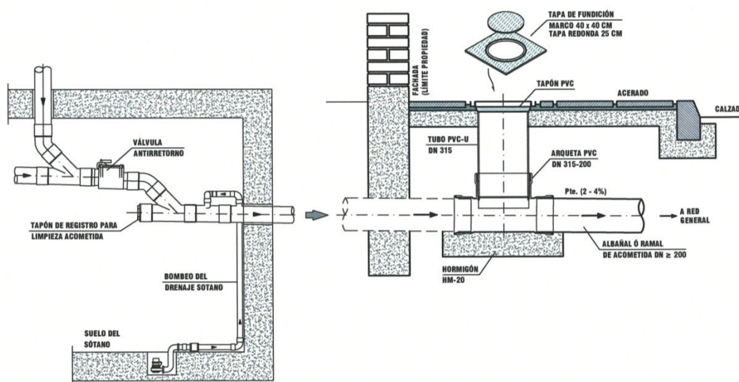
Figura III-3. Edificación con sótano
