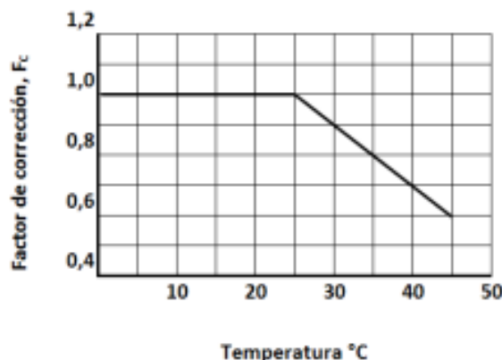
Figura AI-26. Tubos de PVC-U. Factor de corrección de PN por la Tª (UNE-EN 1.456-1)
