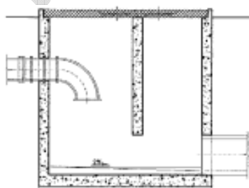
Figura II-7. Cámara de rotura
