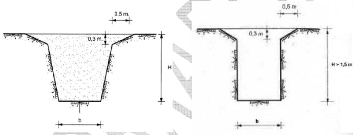
Figura V-1. Bordes ataluzados en zanjas
