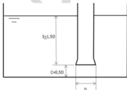
Esquema de sumergencia
