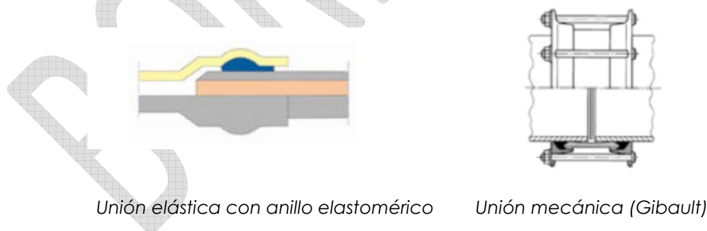
Figura AI-31. Uniones permitidas para los tubos de PVC-U
