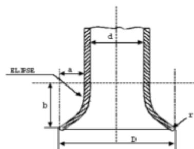
Campana de entrada a tubería de aspiración
